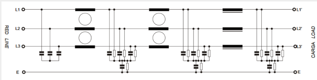
Circuito eléctrico -IT:
