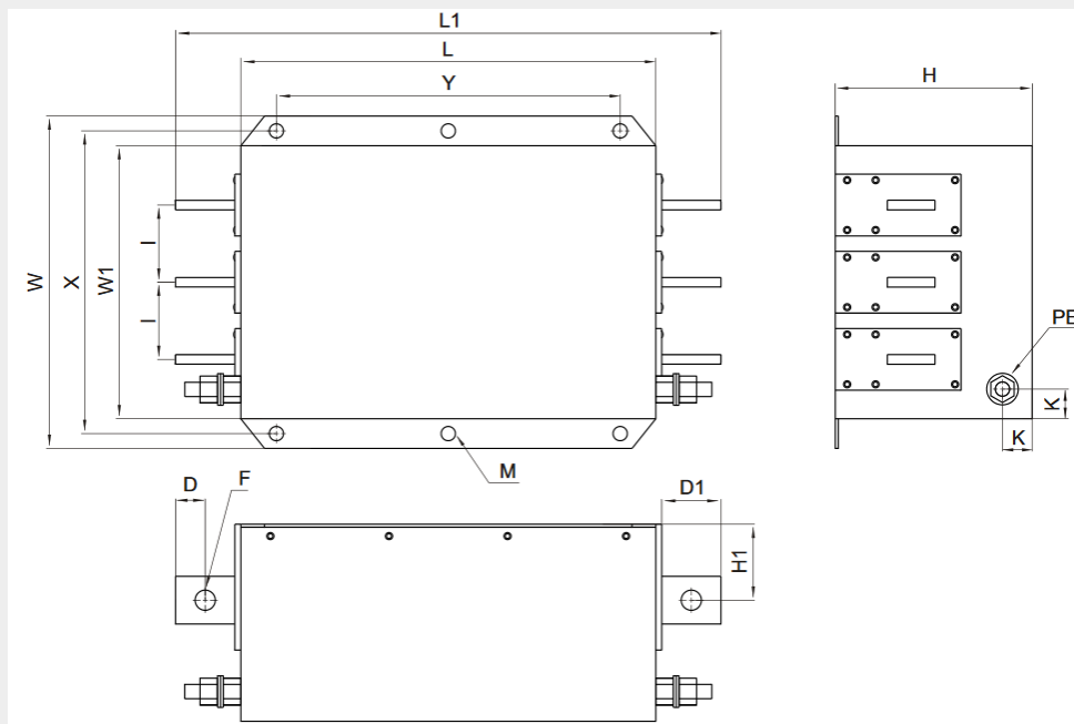
Dimensiones de Cajas Metálicas :
